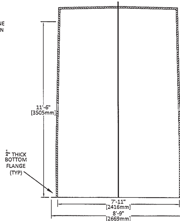
RIGHT ELEV.
