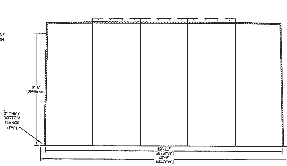
RIGHT ELEV.
