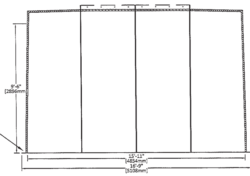
RIGHT ELEV.
