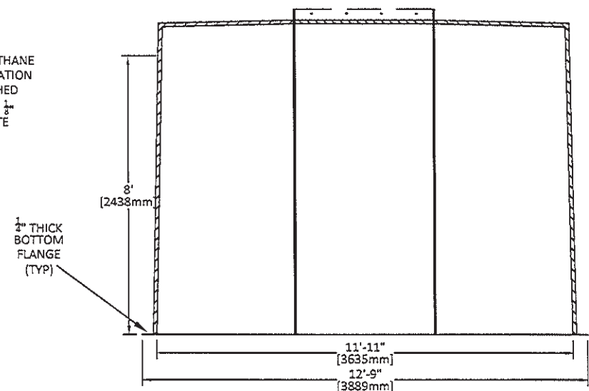
RIGHT ELEV.
