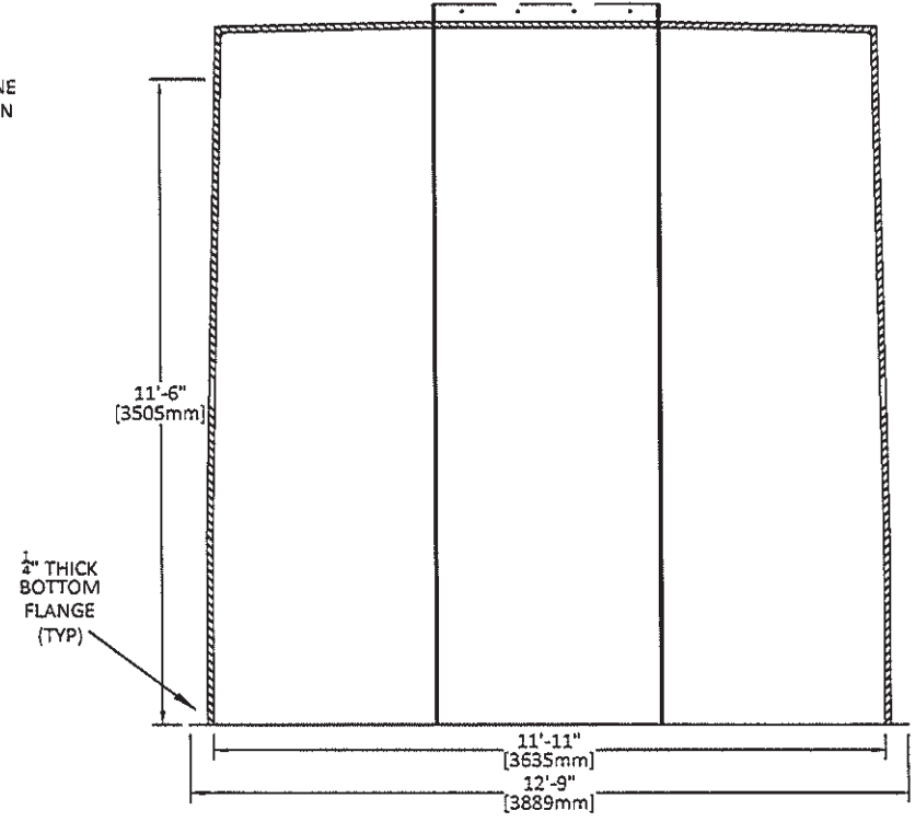
RIGHT ELEV.
